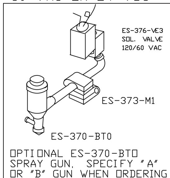
ES-376-VE3 SOL. VALVE 120 / 60 VAC OR 24 VDC
